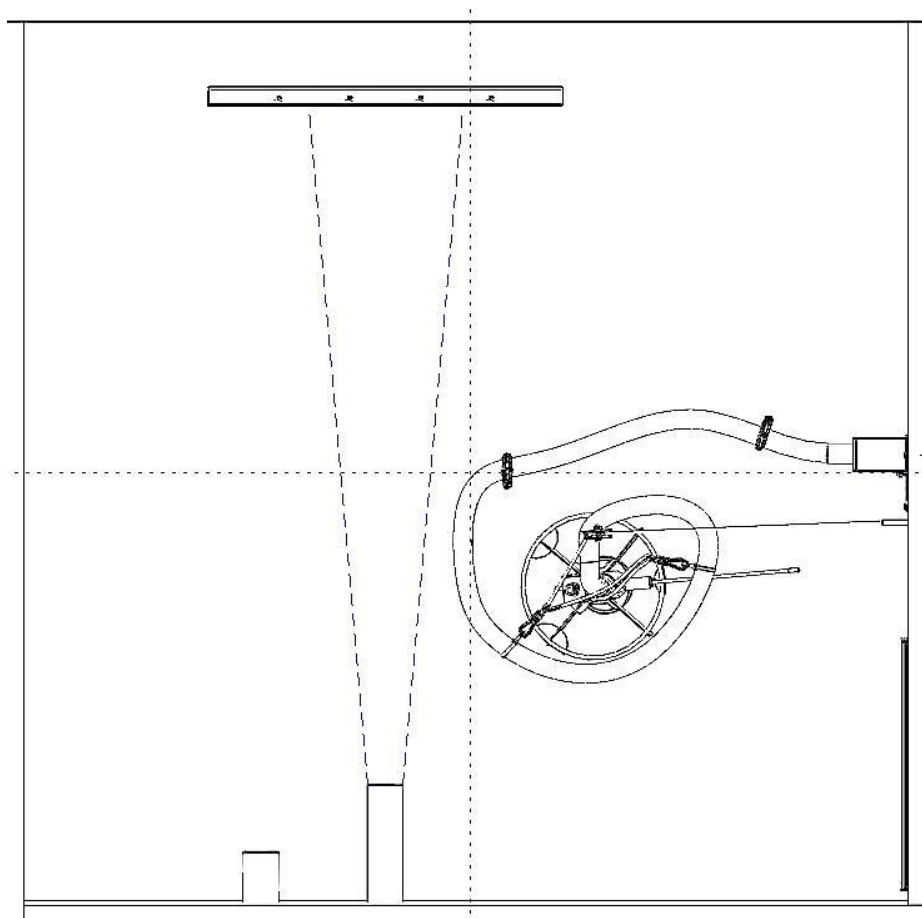
Abbildung 2: Sonnen-Pellet Maulwurf Classic mit Handhebebezug in der Parkposition (Draufsicht)
