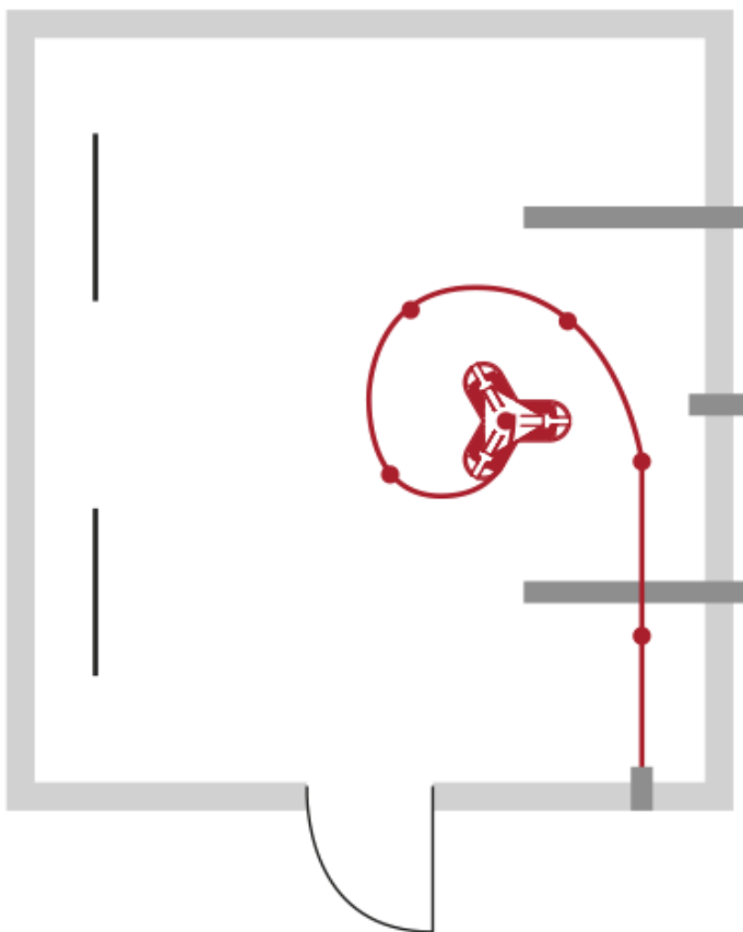
Abbildung 3: Pellet Maulwurf E3 in der Befüllsituation
