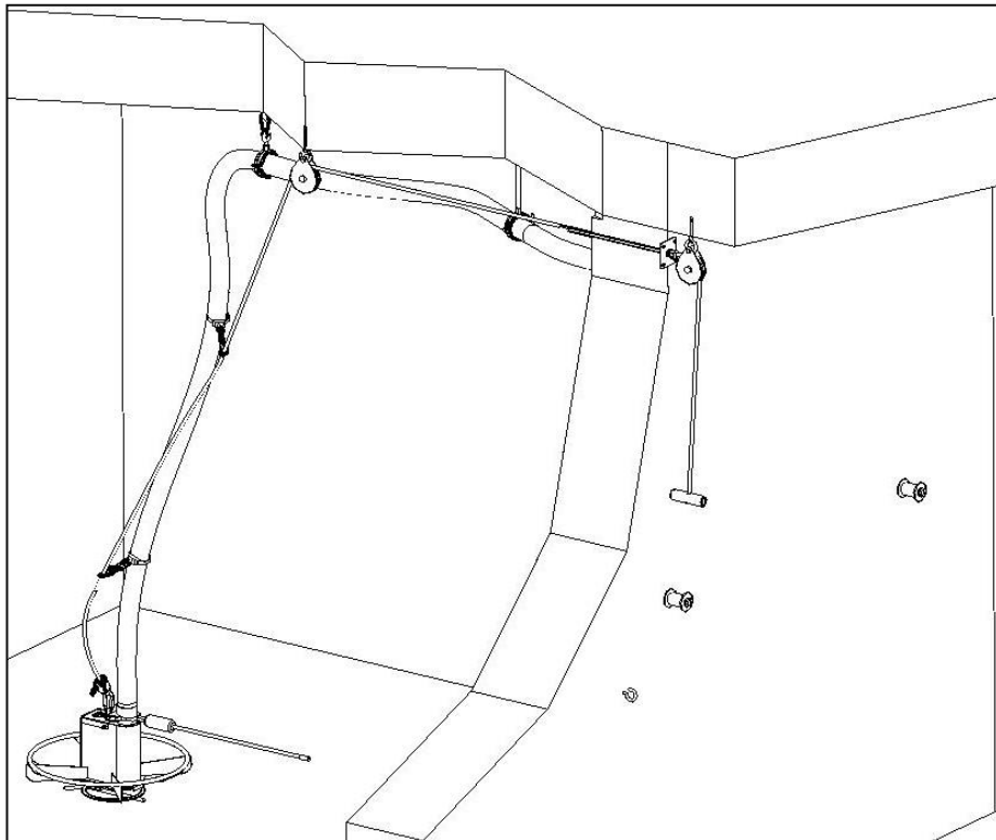
Abbildung 1: Sonnen-Pellet Maulwurf Classic mit Handhebebezug im leeren Lagerraum
