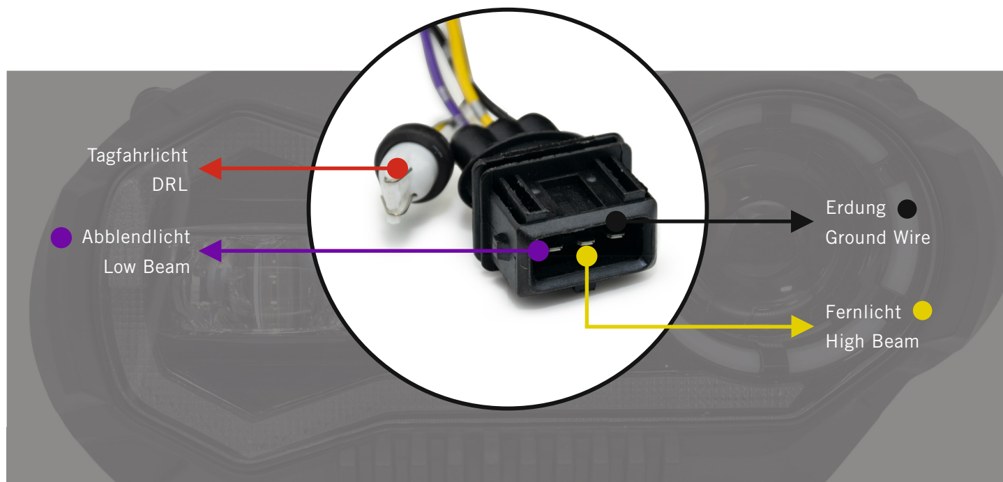
Frontansicht des Scheinwerfers Headlight front view
