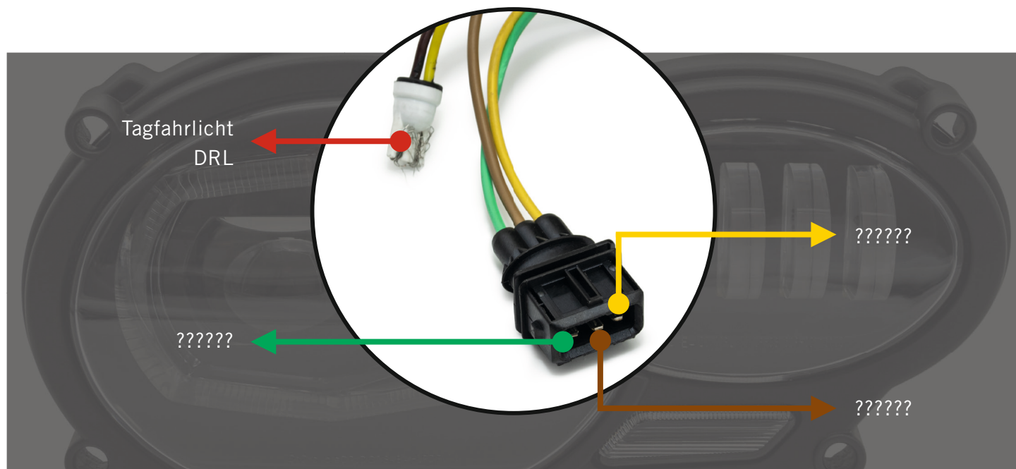
Frontansicht des Scheinwerfers Headlight front view
